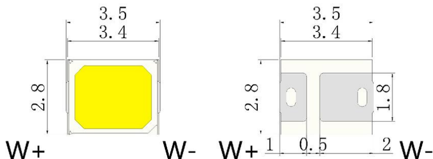
正面图
