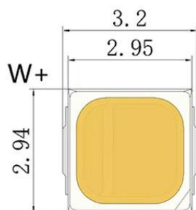
正面图
