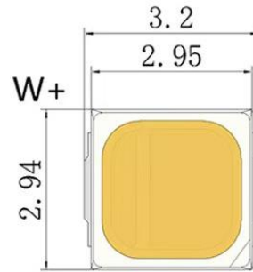
正面图
