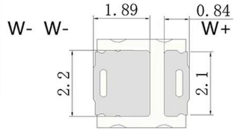
背面图
