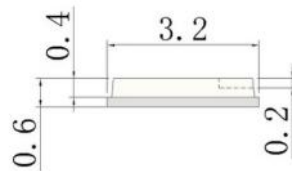
侧面图
