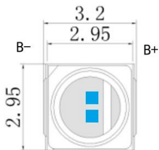
正面图
