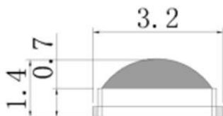
侧面图
