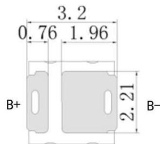
背面图
