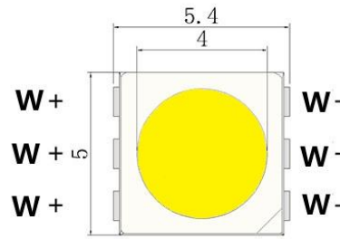
正面图
