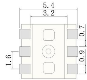
背面图
