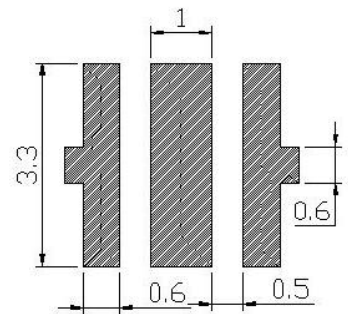
焊盘建议图
