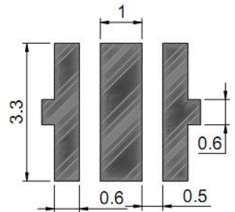
焊盘建议图
