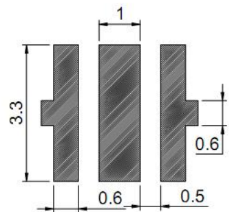
焊盘建议图
