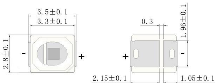
正面图
