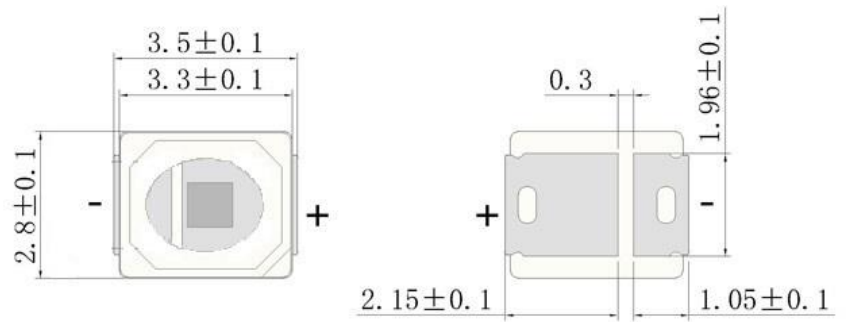
正面图
