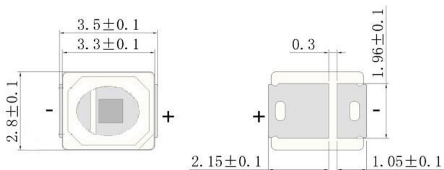
正面图
