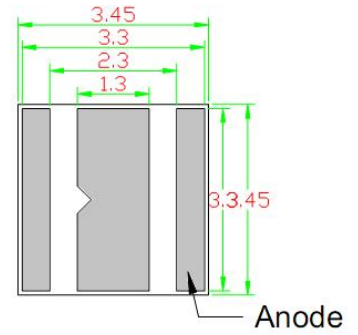
背面图
