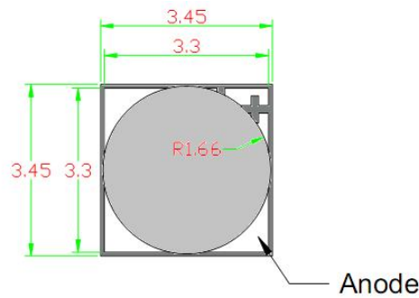
正面图
