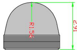
正面图
